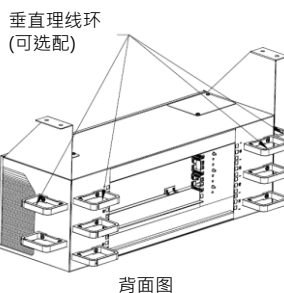
背面图
