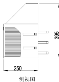
侧视图
