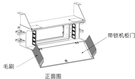
正面图
