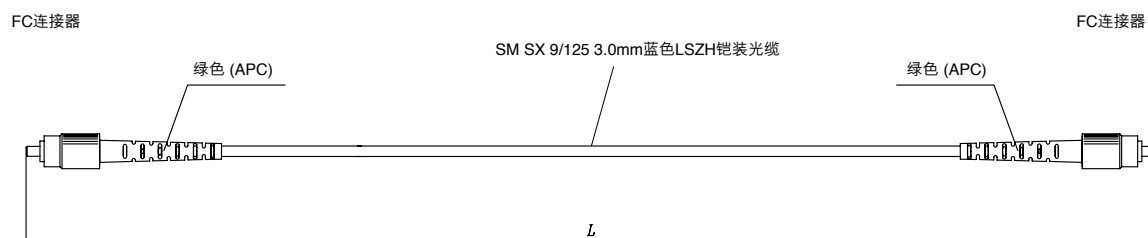
单芯铠装跳线示例—FC-FC，OS1/2，APC，LSZH，5m 产品编号：ARS11AS1L-005M
