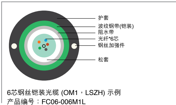
光缆横截面图示
