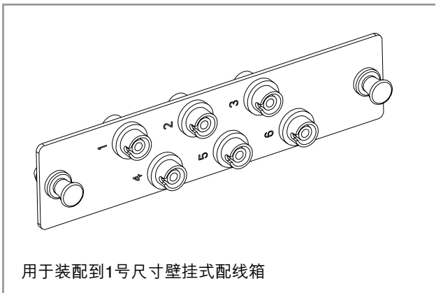
D号尺寸面板：28 (高) x 120 (宽) mm
