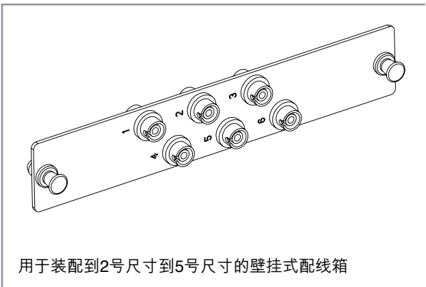
C号尺寸面板：28 (高) x 155 (宽) mm
