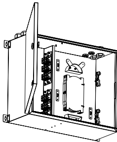
48芯SC熔接示例 产品编号：IWS6-04-Cxxxx
