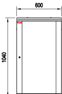
带门正面图
