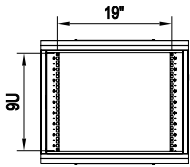
无门正面图
