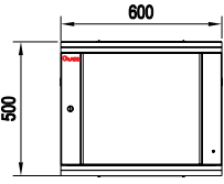
带门正面图
