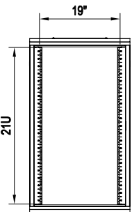
无门正面图
