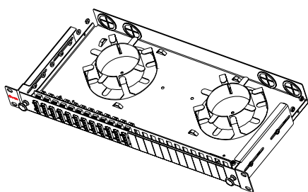
D200示例，LC，48芯，绕线式，OM2 产品编号：R200P1G-4CM2
