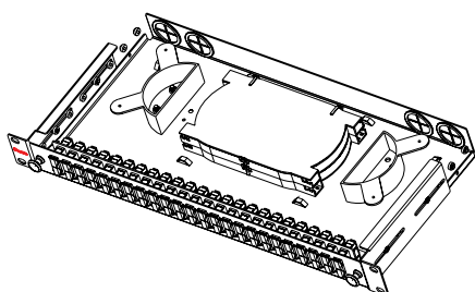
D200示例，SC，48芯，熔接式，OM3 产品编号：R200S1G-2CM3
