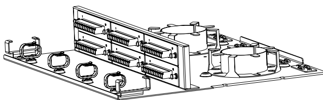
带有6插槽的2U绕线式抽屉 用于容纳6套B号尺寸面板 (参见第112页)
