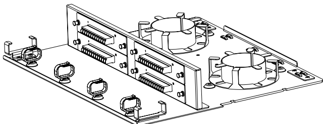
带有4插槽的2U绕线式抽屉 用于容纳4套A号尺寸面板 (参见第112页)
