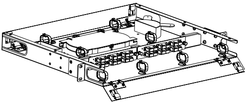
1U固定式光纤配线箱 (水平式)
