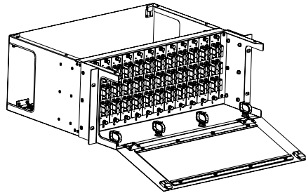
4U固定式光纤配线箱 (垂直式)
